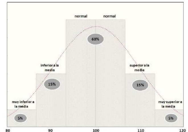
Figura 2: Ejemplo de distribución de los valores genéticos
